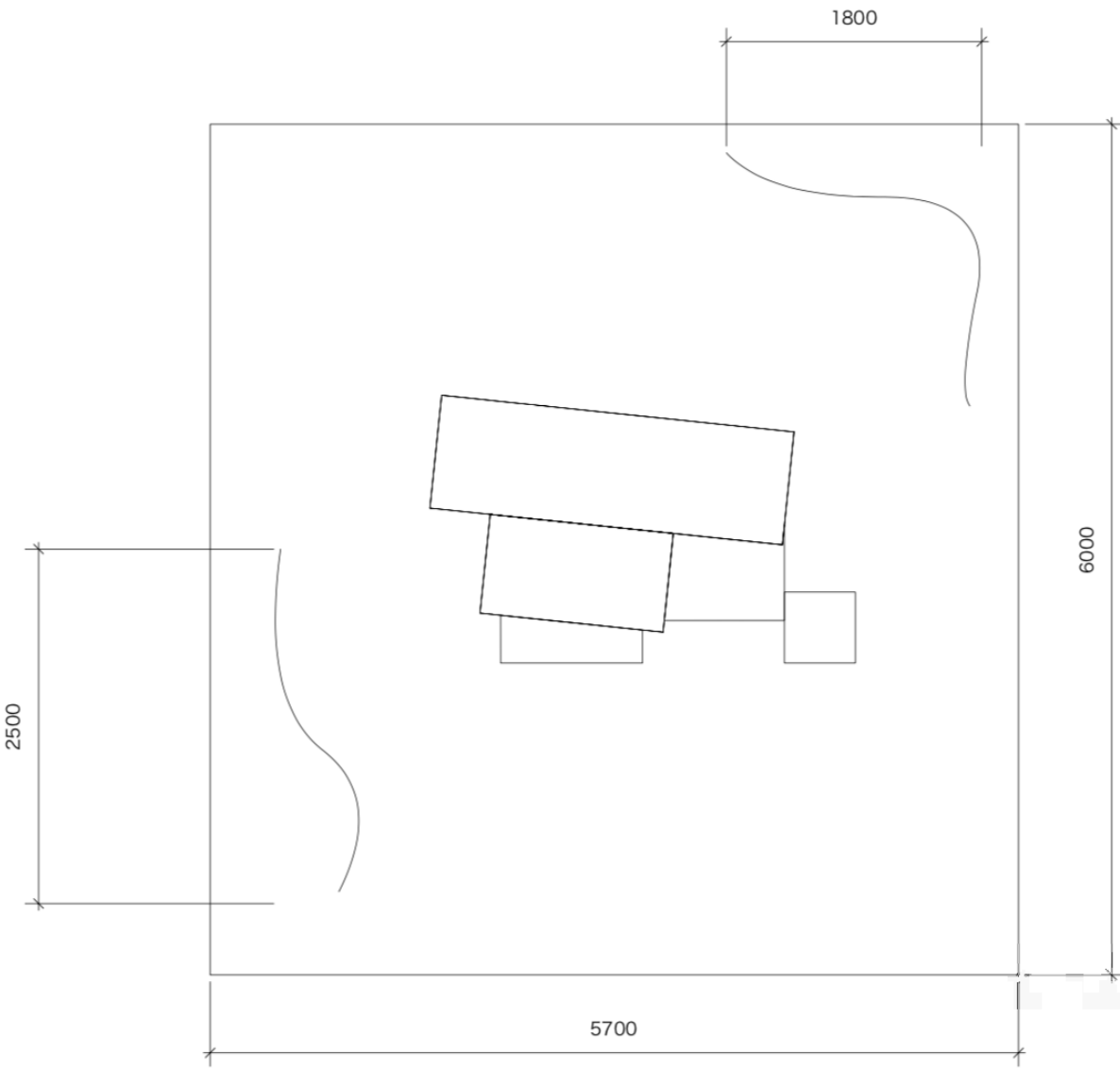
1/30 平面図
